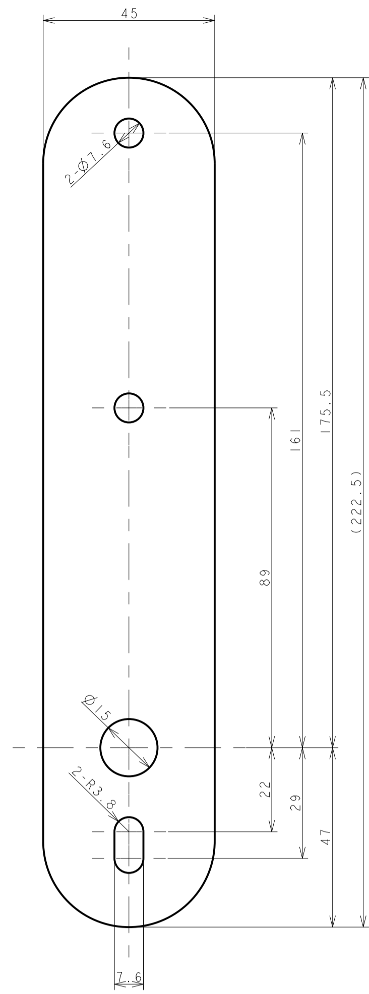
ロックベーススペーサー 厚み 1.0mm / 2.0mm / 3.0mm
