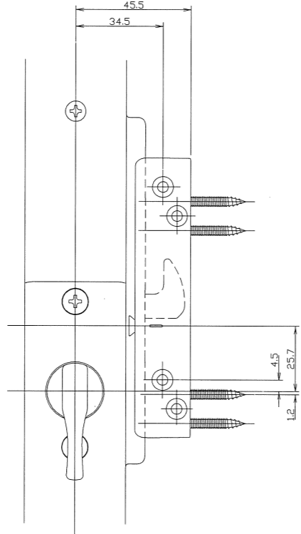
面付受取収まり図
