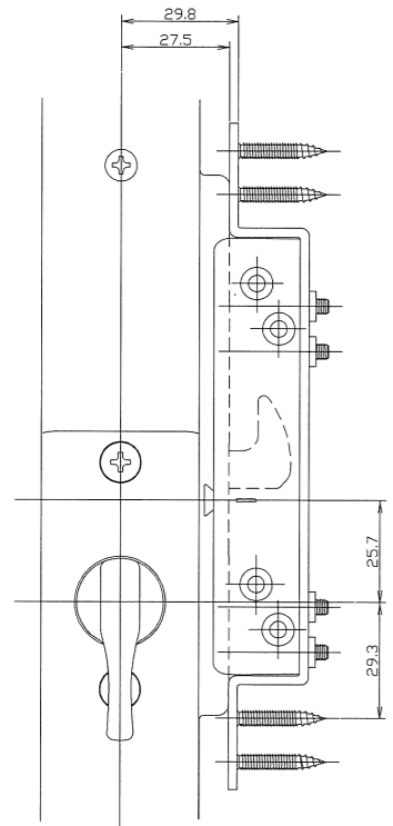
据込み受取収まり図
