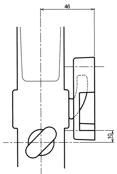
受箱 (B) 納まり図
